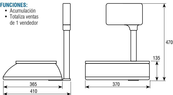
Dimensiones (mm)
