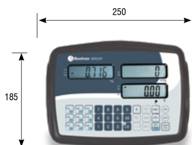
Dimensiones (mm)
